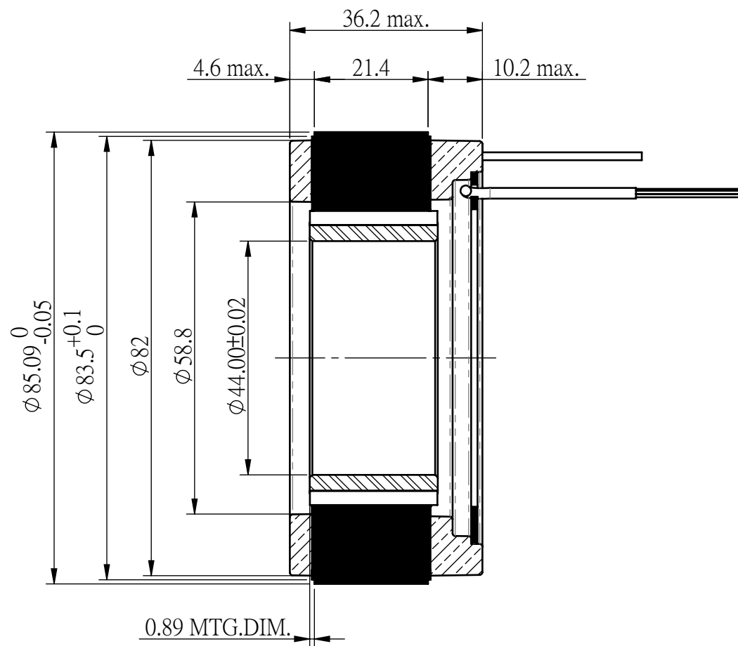
剖面圖 A-A
