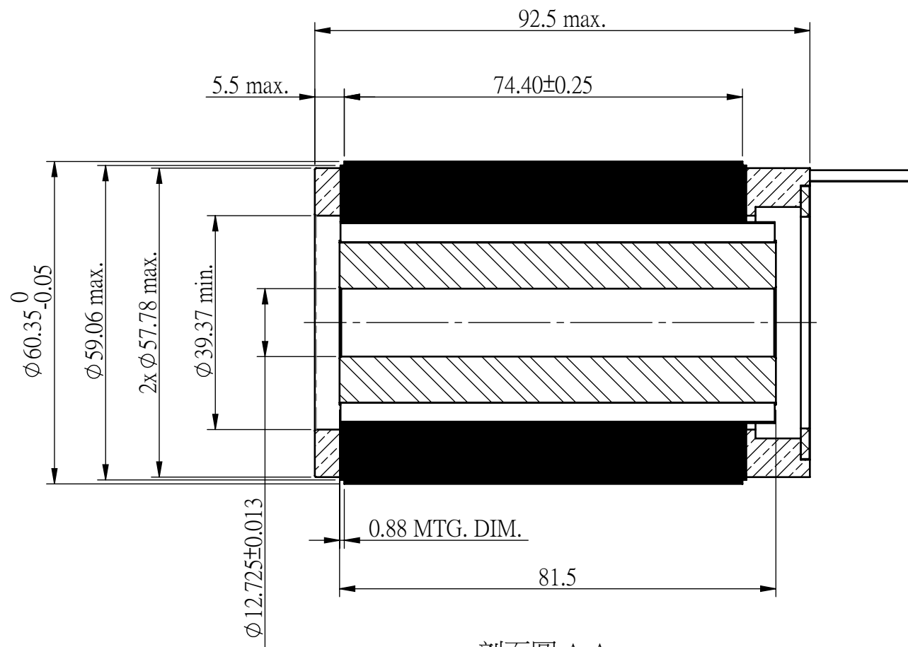
剖面圖 A-A
