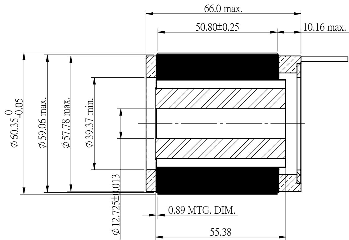
剖面圖 A-A
