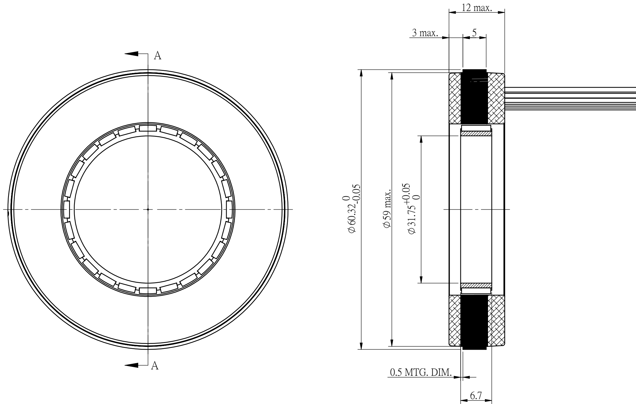
剖面圖 A-A
