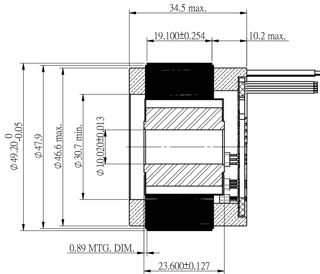
剖面圖 A-A
