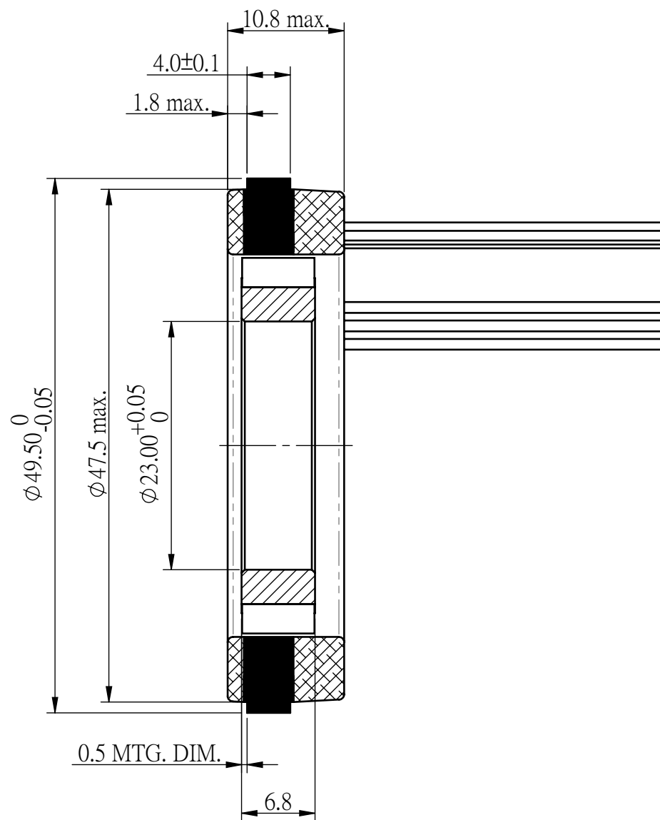
剖面圖 A-A
