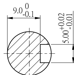
剖面圖 A-A 比例 2:1
