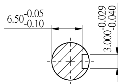
剖面圖 A-A 比例 2 : 1
