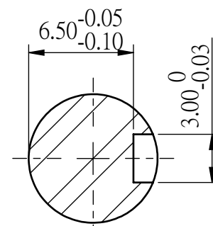
剖面圖 A-A 比例 3 : 1
