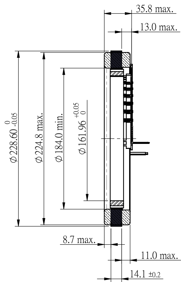
剖面圖 A-A
