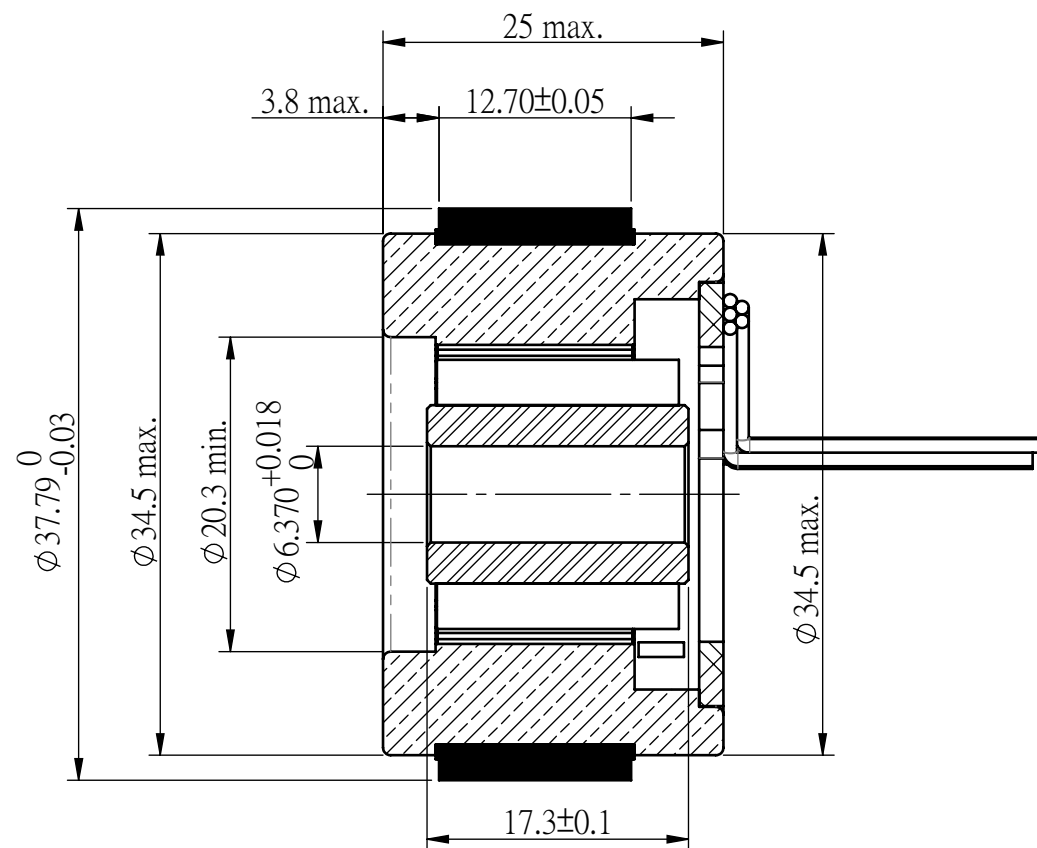
剖面圖 A-A
